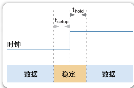
► 图10. 数字信号的建立时间和保持时间定义。
