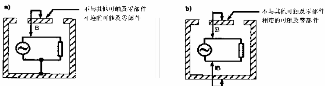
图 D.2a) 和 D.2b) 不与其他可触及零部件相连的可触及件对内部危险带电电路的防护
