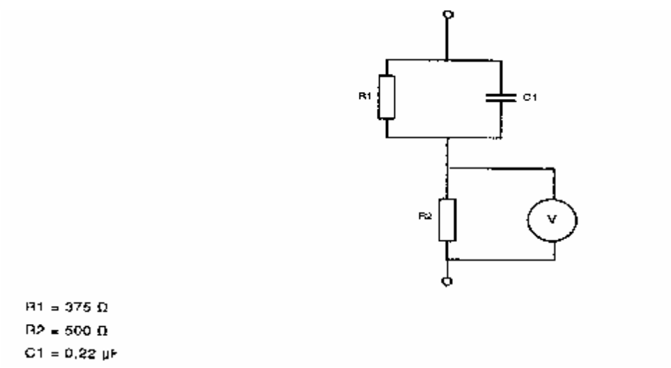
图 A.4 潮湿接触电流测量电路
