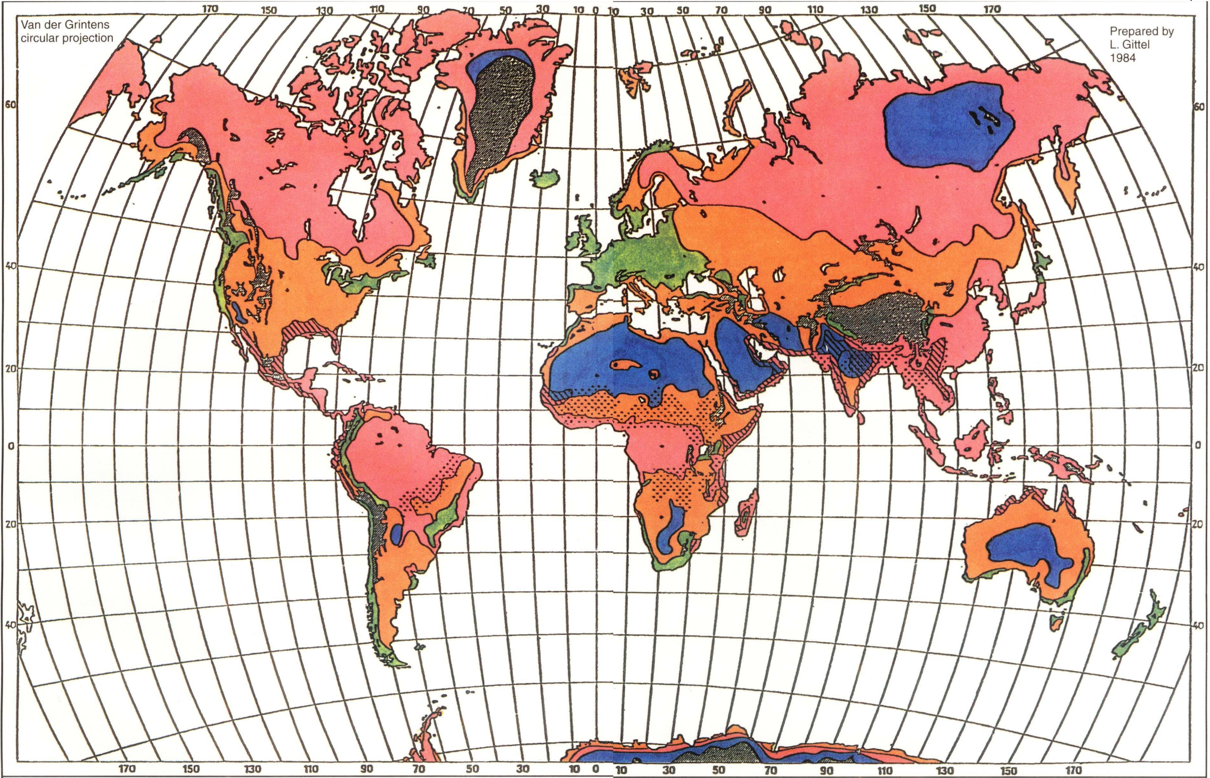
图 A.2 洲和大的岛屿的户外气候 IEC 标准 721-2-1: 自然环境条件 温度和湿度
