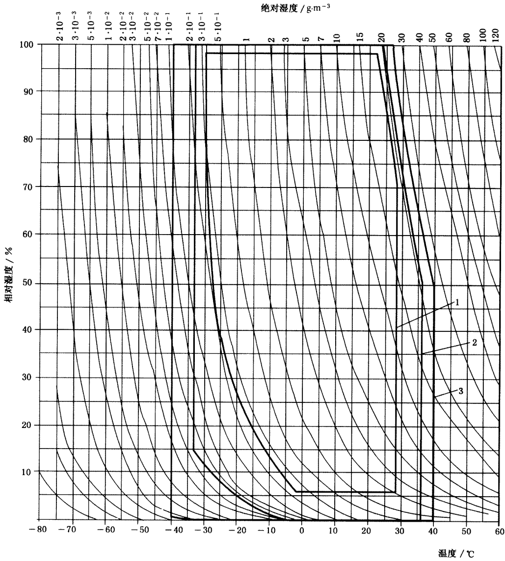
图 11 统计的户外气候——寒温 I (仅适用于中国)
