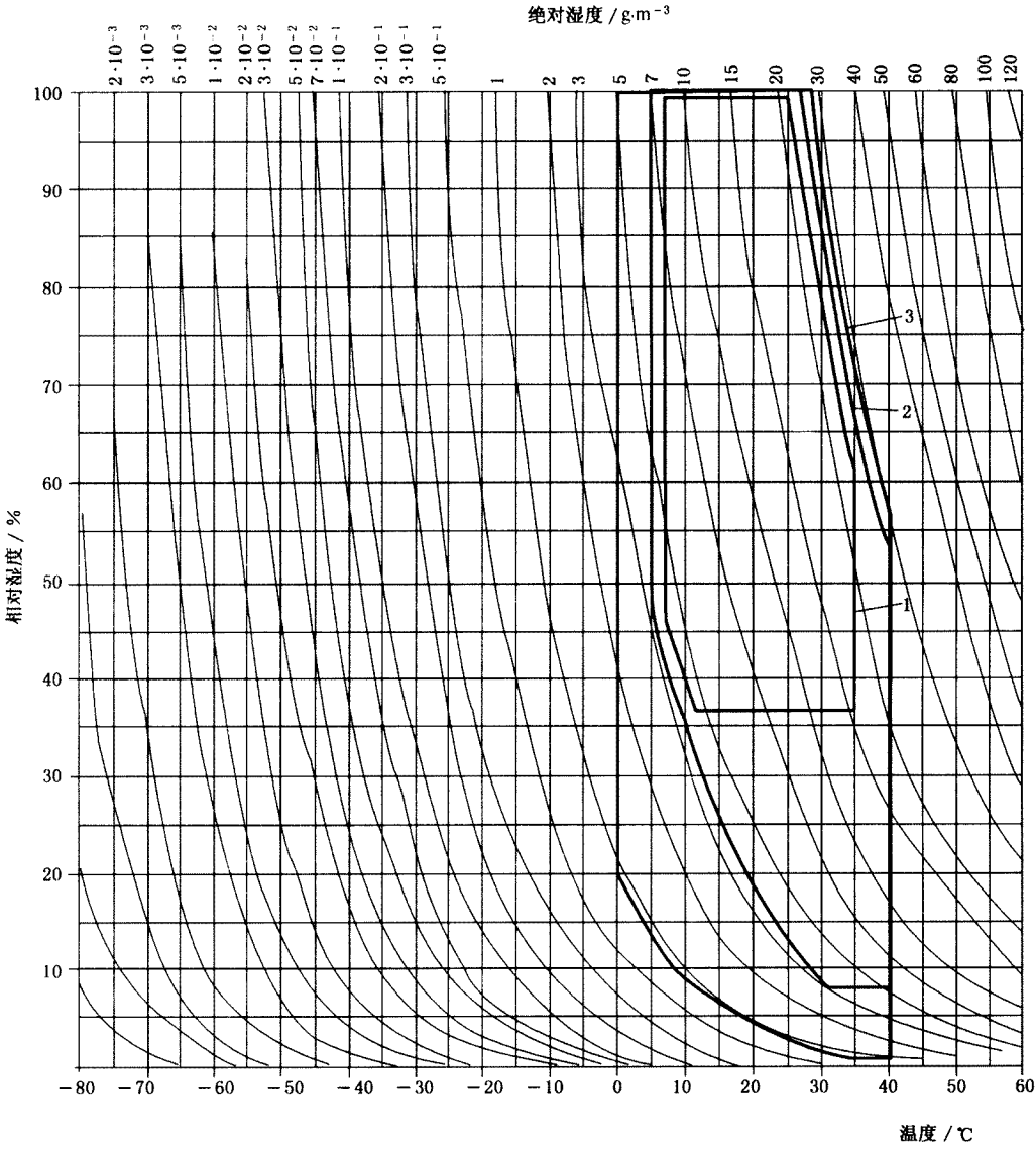
图 16 统计的户外气候——湿热 (仅适用于中国)
