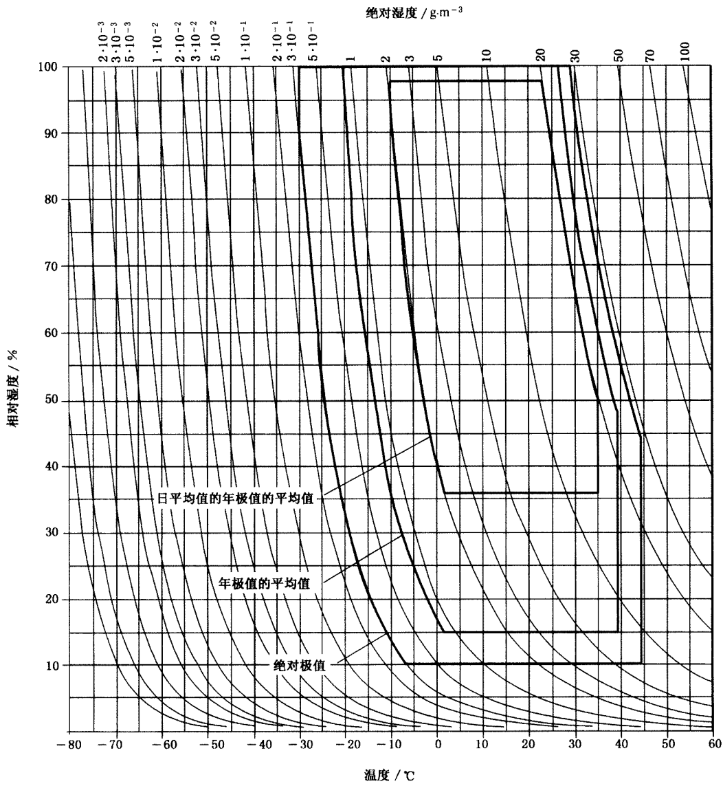
图 5 统计的户外气候——干热
